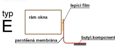
Flexi tesniaci okenní pás INTERIÉR
