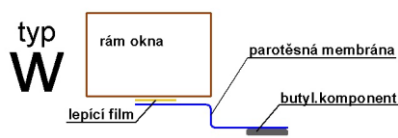
Flexi tesniaci okenní pás EXTERIÉR
